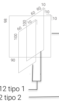
Schema montaggio staffe
