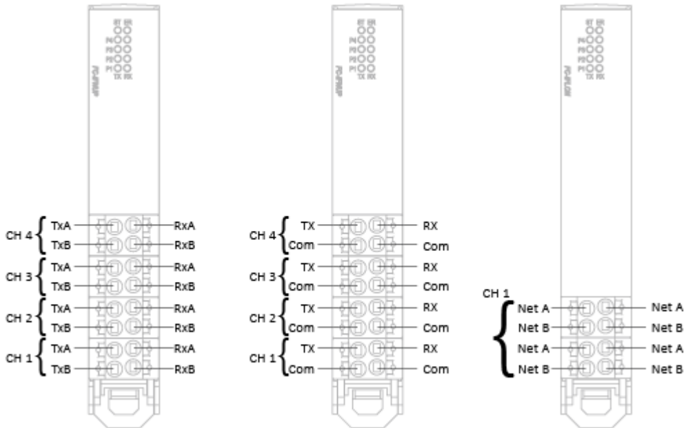
Modulo Nuovo Pignone
