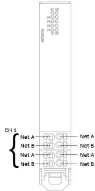
Cablaggio Periferiche (Erogatore, Centraline, Prezziari)
